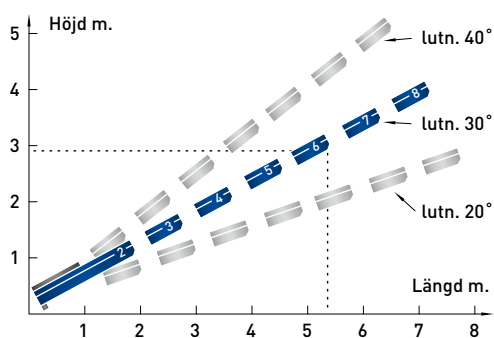
Höjd/längd diagram
